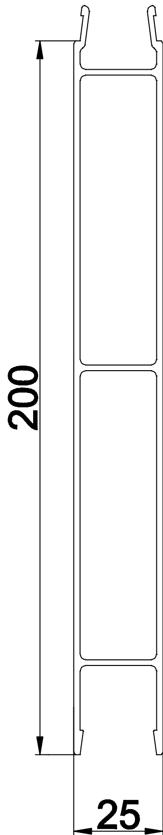
Profil 5021 200 mellemprofil L: 5100 mm + 6600 mm vægt: 2,36 kg/m
